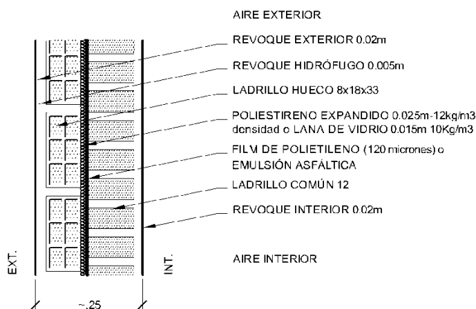
MURO DOBLE LADRILLO COMUN DE 12/HUECO DE 8 + AISLACION (7 CAPAS) K=0.76 W/m²K
