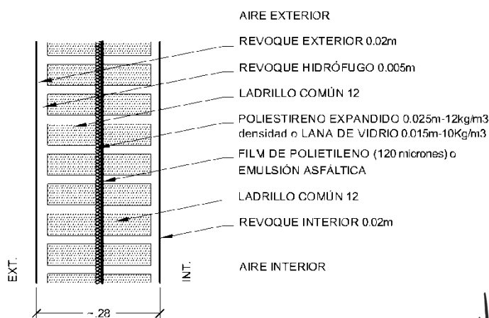
MURO DOBLE + AISLACION LADRILLO COMUN DE 12 (7CAPAS) K=0.57 W/m²K
