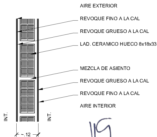
MURO DE LADRILLO CERAMICO HUECO DE 8x18x33 Arq. Miguel G. Garaycochea Director General de Planificación Territorial Municipalidad de Berazategui
